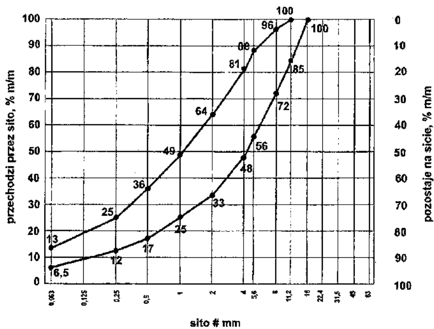
Rys. 4. Krzywe graniczne uziarnienia mieszanki mineralnej 0/1,2 mm
